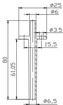
图 5: 连接件 1003
