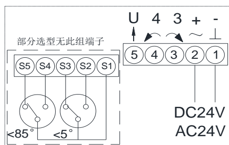
端子接线图
