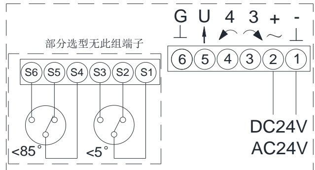
端子接线图
